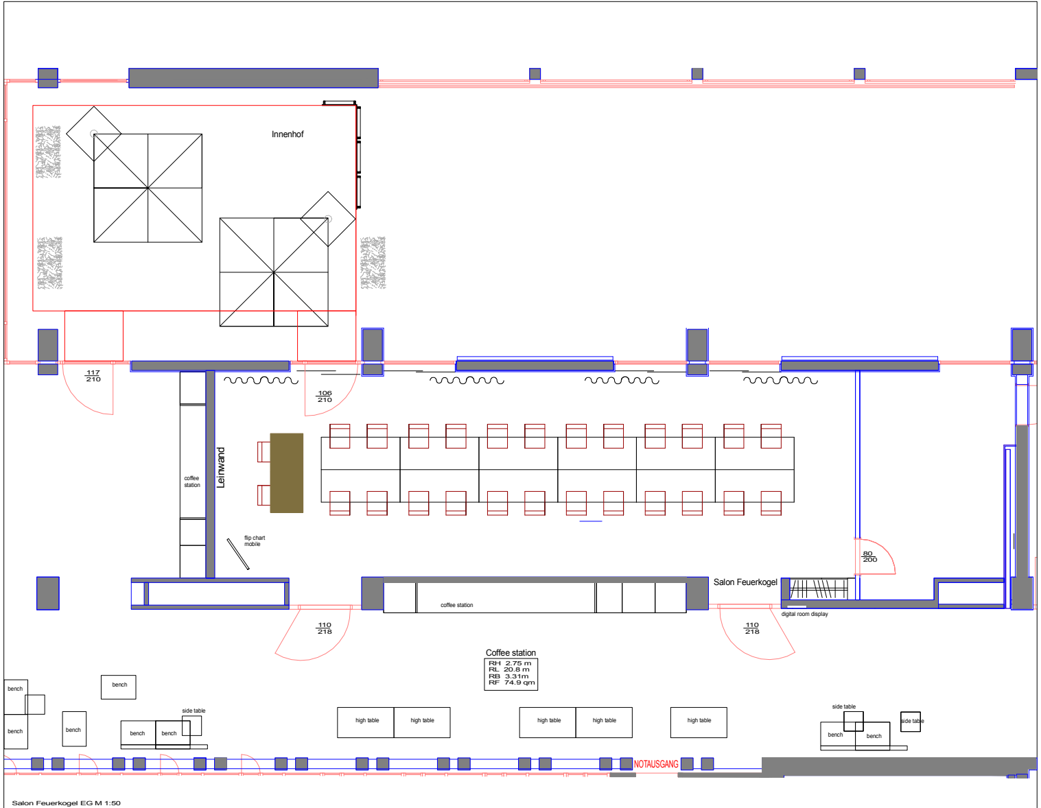
Salon Feuerkogel EG M 1:50
